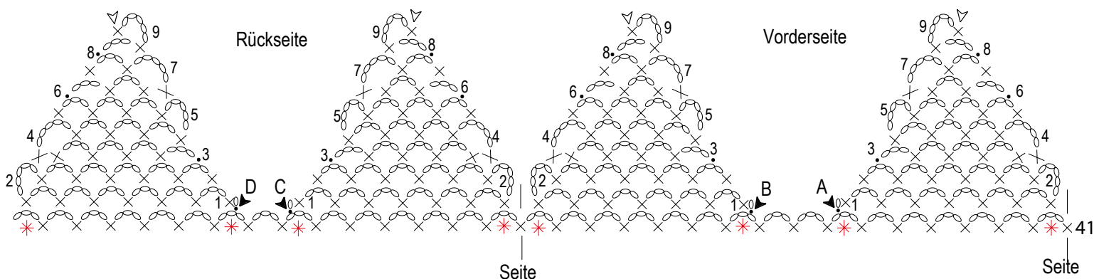
Schema 2: Obere dreieckige Motive
